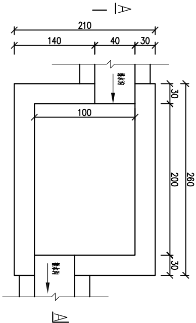
沉沙池平面图
